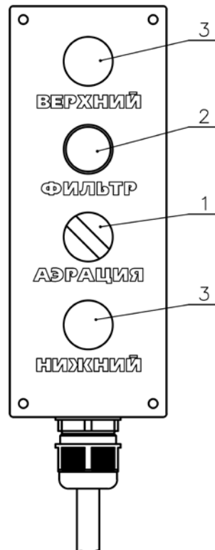
Рис.6. Пульт выносной
